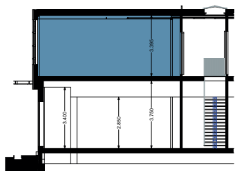
Doorsnede A-A
